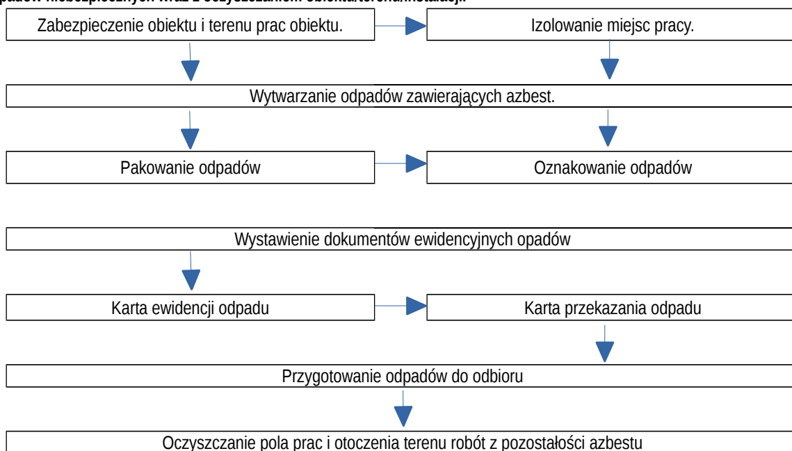
Rysunek 5. Schemat procedury dotyczącej prac polegających na usuwaniu wyrobów zawierających azbest, wytwarzania odpadów niebezpiecznych wraz z oczyszczaniem obiektu/terenu/installacji.
